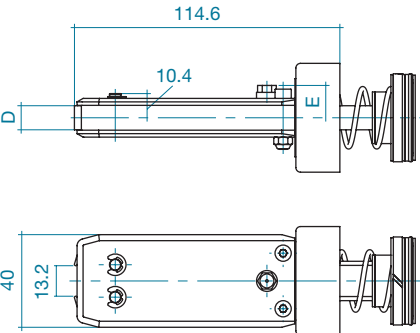
延伸 42 mm, 窄
